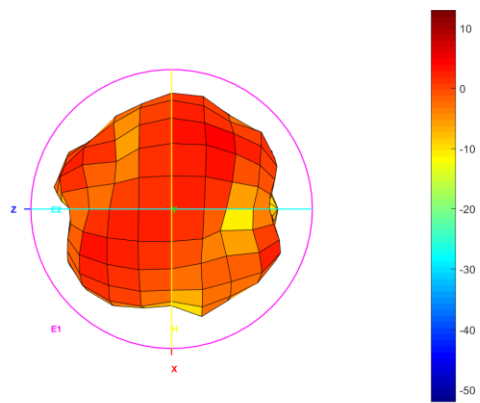
Total_3D_Left View_5.8GHz
