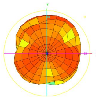
Total_3D_Side View_1_1.71GHz
