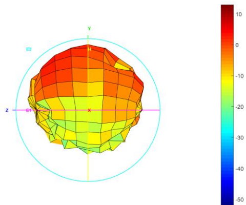
Total_3D_Left View_5.8GHz
