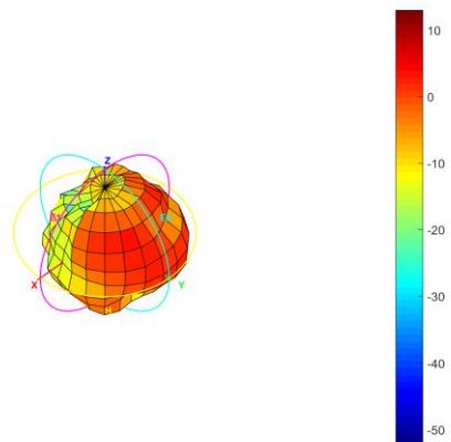
Total_3D_Side View 1_5.8GHz
